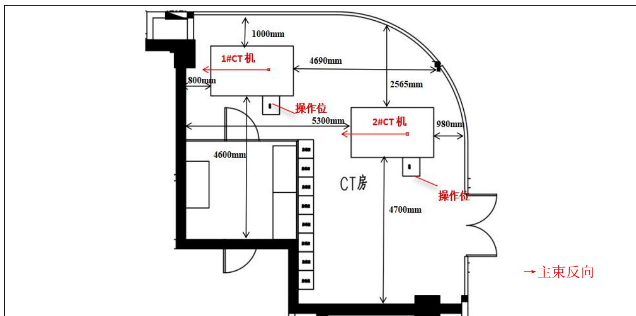
图 11-1 工业 CT 机的摆放位置图
