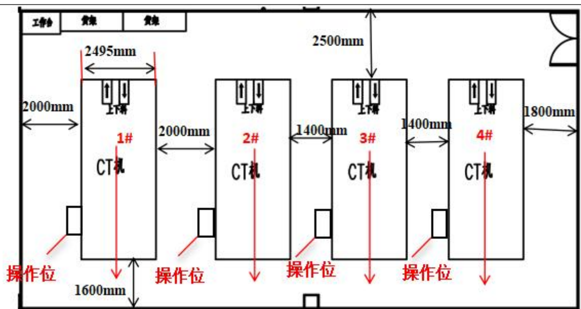
图 1.3-13 W1 厂房 CT 检测区平面布置图
