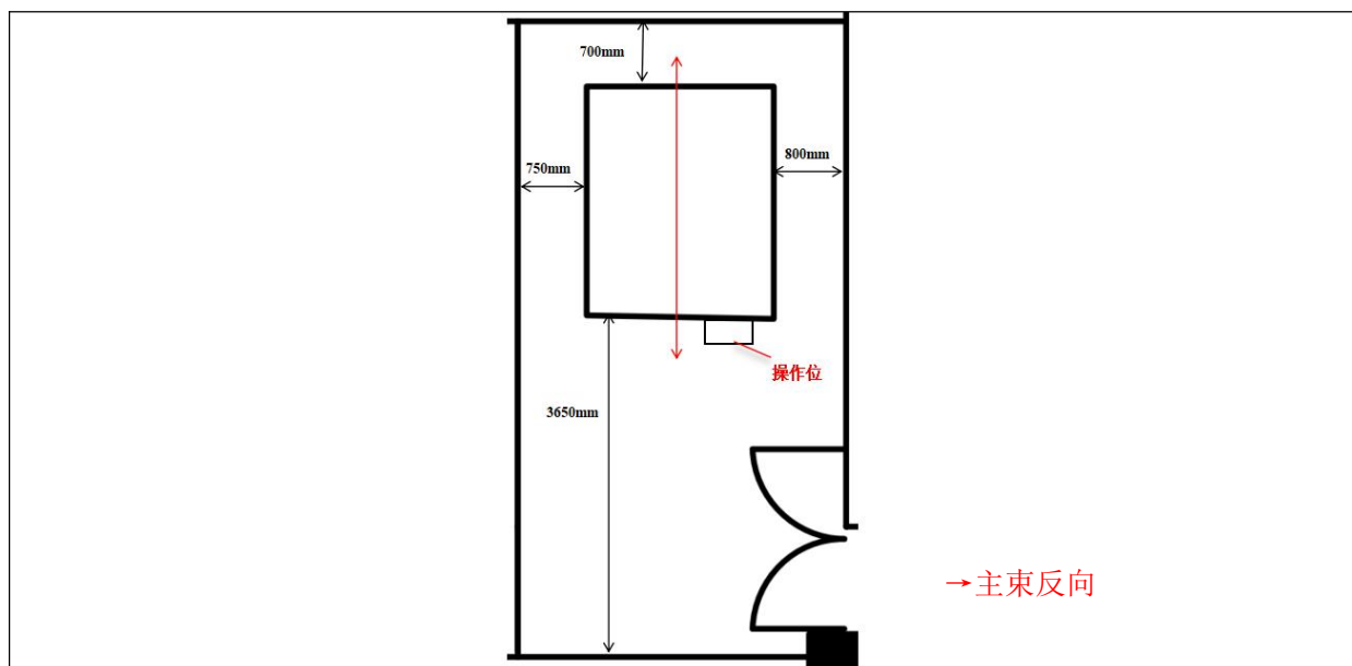
图 11-2 M2 厂房 CT 室的摆放位置图
