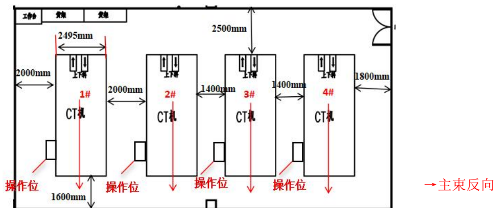
图 11-3 W1 厂房 CT 检测区的摆放位置图
