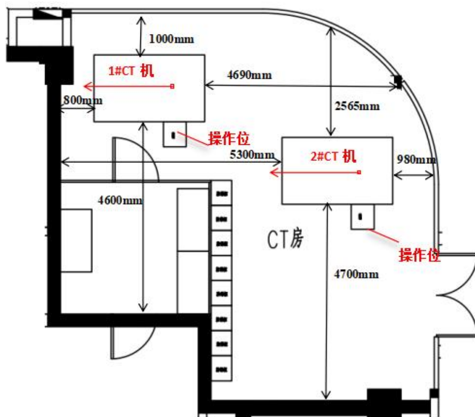
图 1.3-3 3 号 CT 室平面布置图
