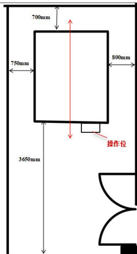
图 1.3-8 M2 厂房 CT 室平面布置图
